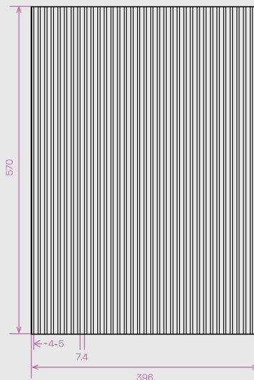
LAMEL KRAFT 3 technický náčrt
