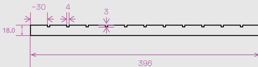
LAMEL PRIME 1 technický náčres
