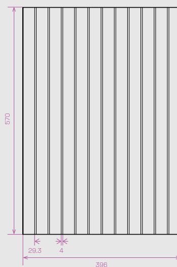
LAMEL PRIME 1 technický náčres
