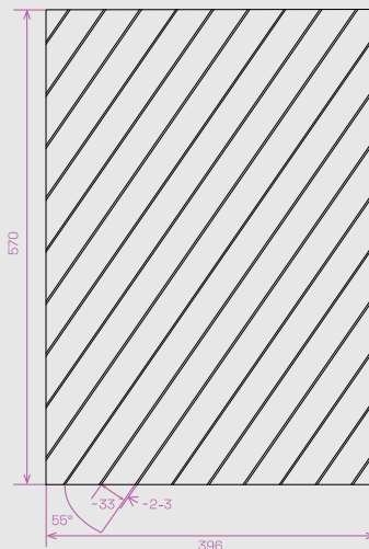
LAMEL KRAFT 6 technický náčres
