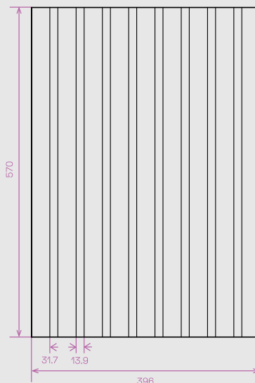
LAMEL KRAFT 2 technický náčrt
