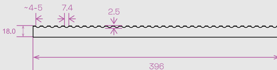
LAMEL KRAFT 3 technický náčrt
