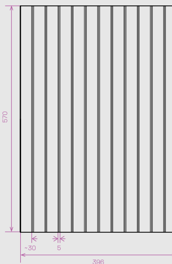
LAMEL VALUE 1 technický nákres
