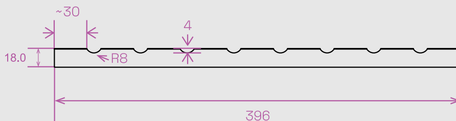
LAMEL KRAFT 2 technický náčrt
