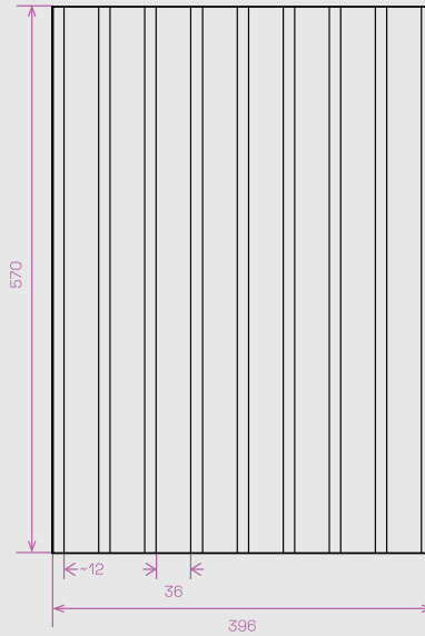
LAMEL KRAFT 4 technický nákres
