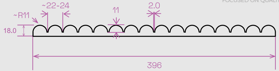
LAMEL BEND 24 prierez
