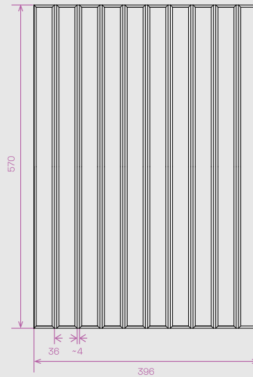
LAMEL VALUE 2 technický náčrt
