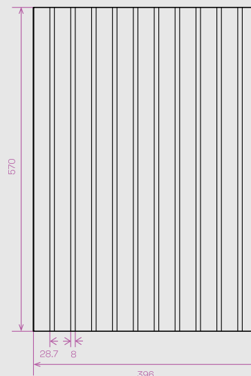
LAMEL KRAFT 1 technický náčrt
