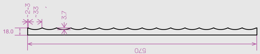
LAMEL KRAFT 5 technický nákres
