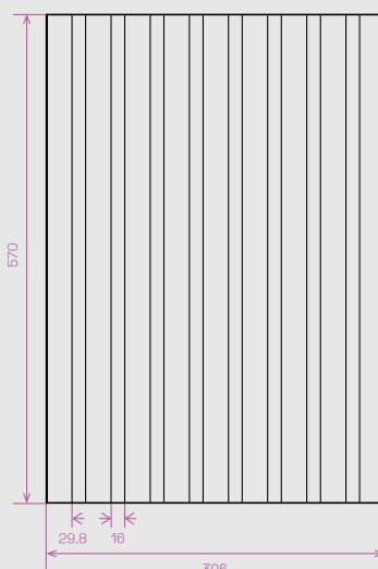
LAMEL PRIME 2 technický nákres
