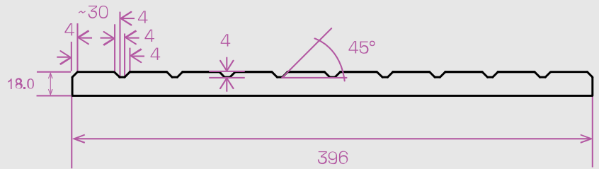
LAMEL VALUE 2 technický náčrt
