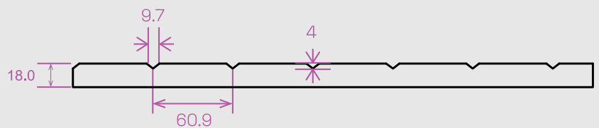
LAMEL VALUE 3 technický náčrt
