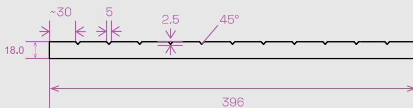
LAMEL VALUE 1 prierez
