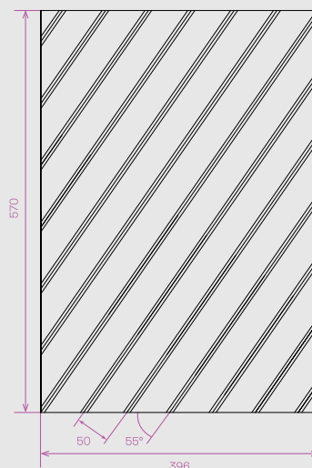
LAMEL VALUE 3 technický náčrt
