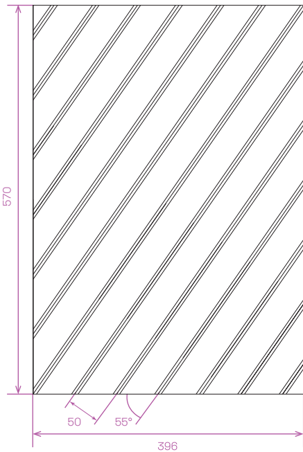
LAMEL VALUE 3 technický nákres
