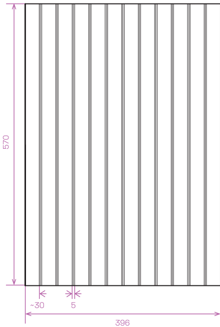
LAMEL VALUE 1 technický náčrt
