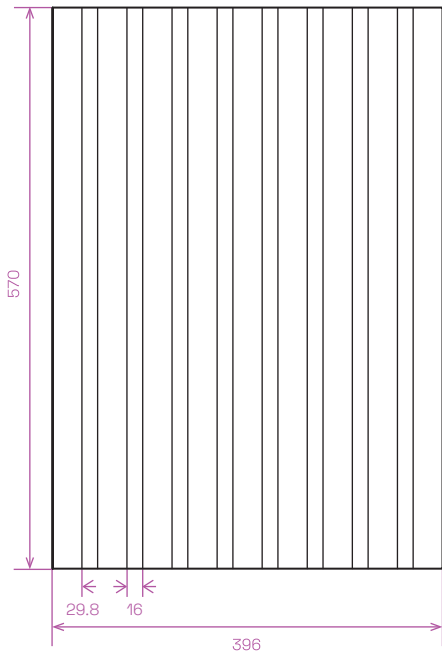
LAMEL PRIME 2 technický náčrt
