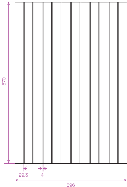
LAMEL PRIME 1 technický náčrt
