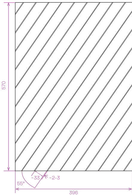
LAMEL KRAFT 6 technický náčres
