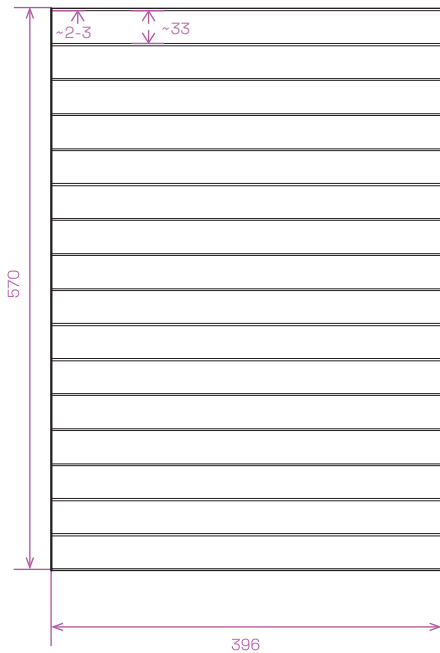
LAMEL KRAFT 5 technický náčrt
