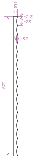
LAMEL KRAFT 5 prierez
