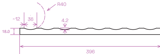
LAMEL KRAFT 4 prierez
