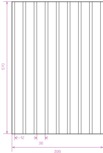
LAMEL KRAFT 4 technický náčrt
