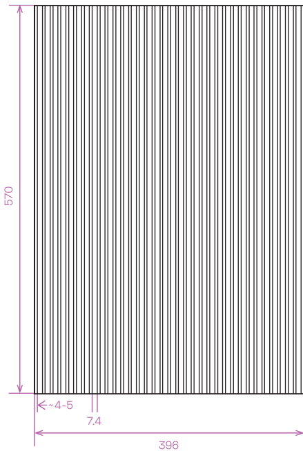
LAMEL KRAFT 3 technický náčrt
