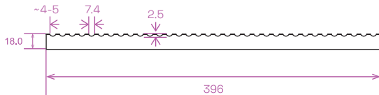
LAMEL KRAFT 3 prierez
