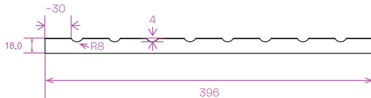
LAMEL KRAFT 2 prierez
