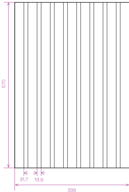
LAMEL KRAFT 2 technický náčrt
