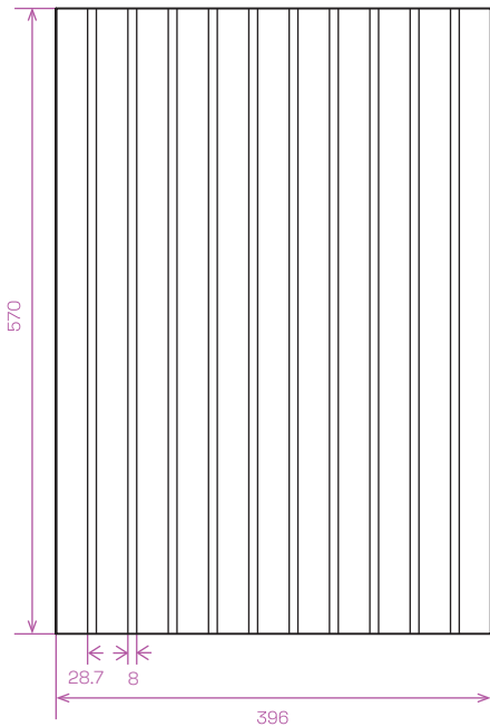
LAMEL KRAFT 1 technický náčrt
