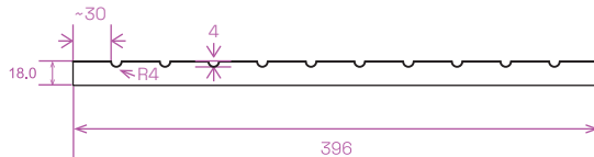
LAMEL KRAFT 1 prierez
