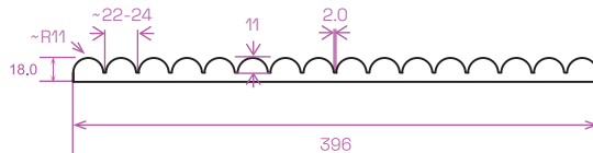
LAMEL BEND 24 prierez
