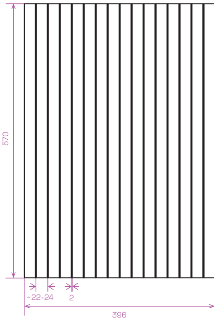
LAMEL BEND 24 technický nákres
