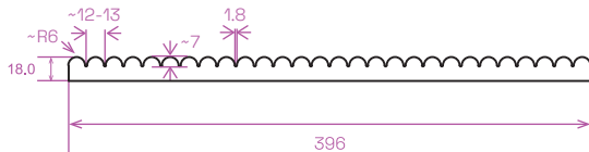
LAMEL BEND 12 prierez
