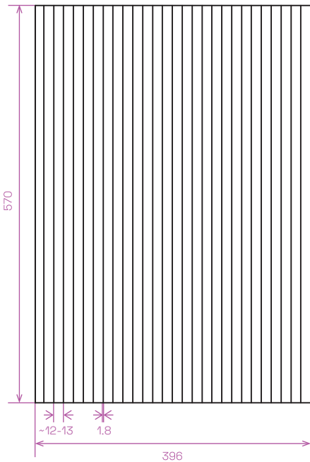
LAMEL BEND 12 technický náčrt
